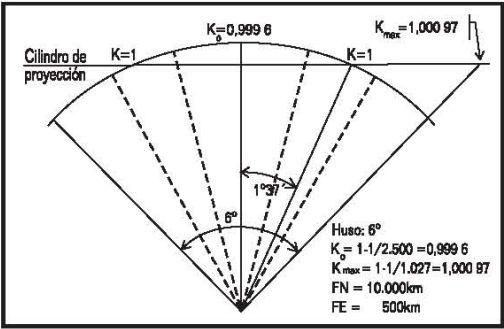
Figura 3 - Proyección UTM
